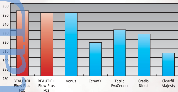
Предел прочности на сжатие в МПа
